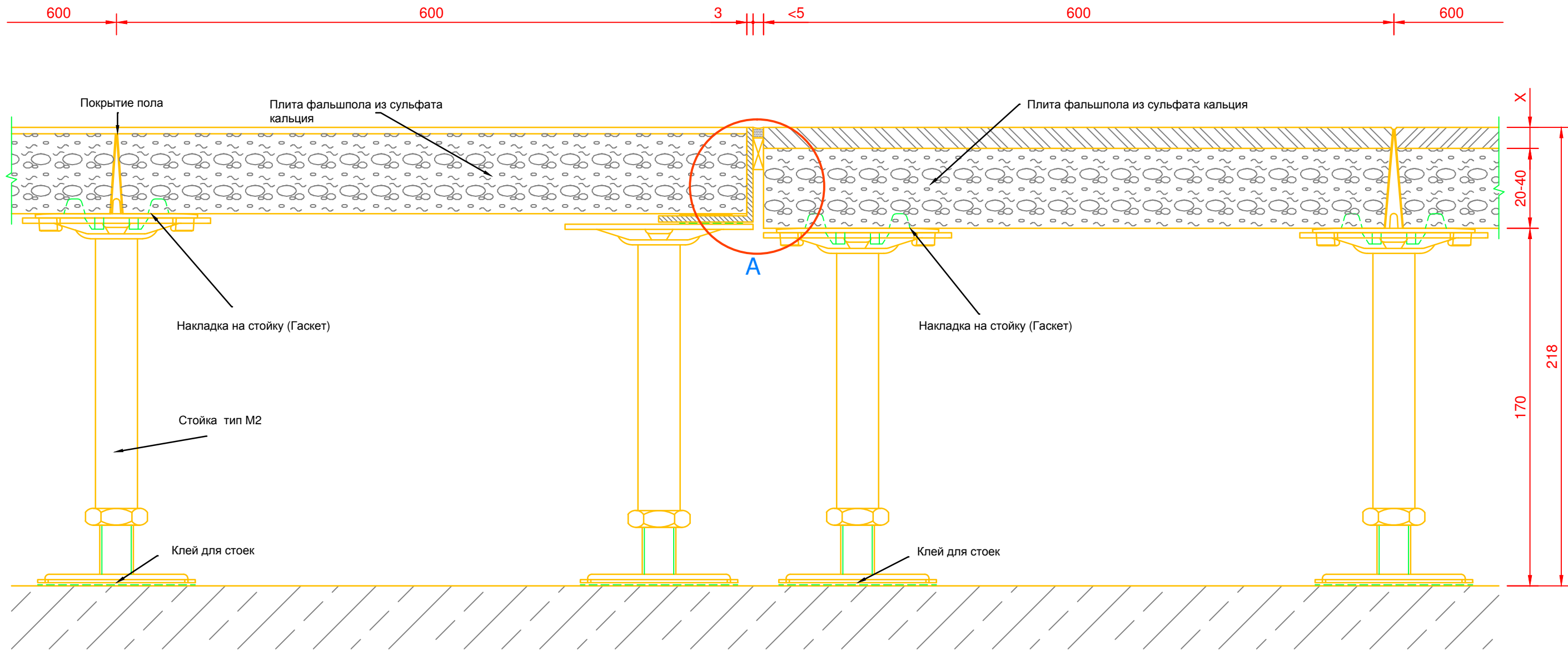
DETAIL A Масштаб 1:1
